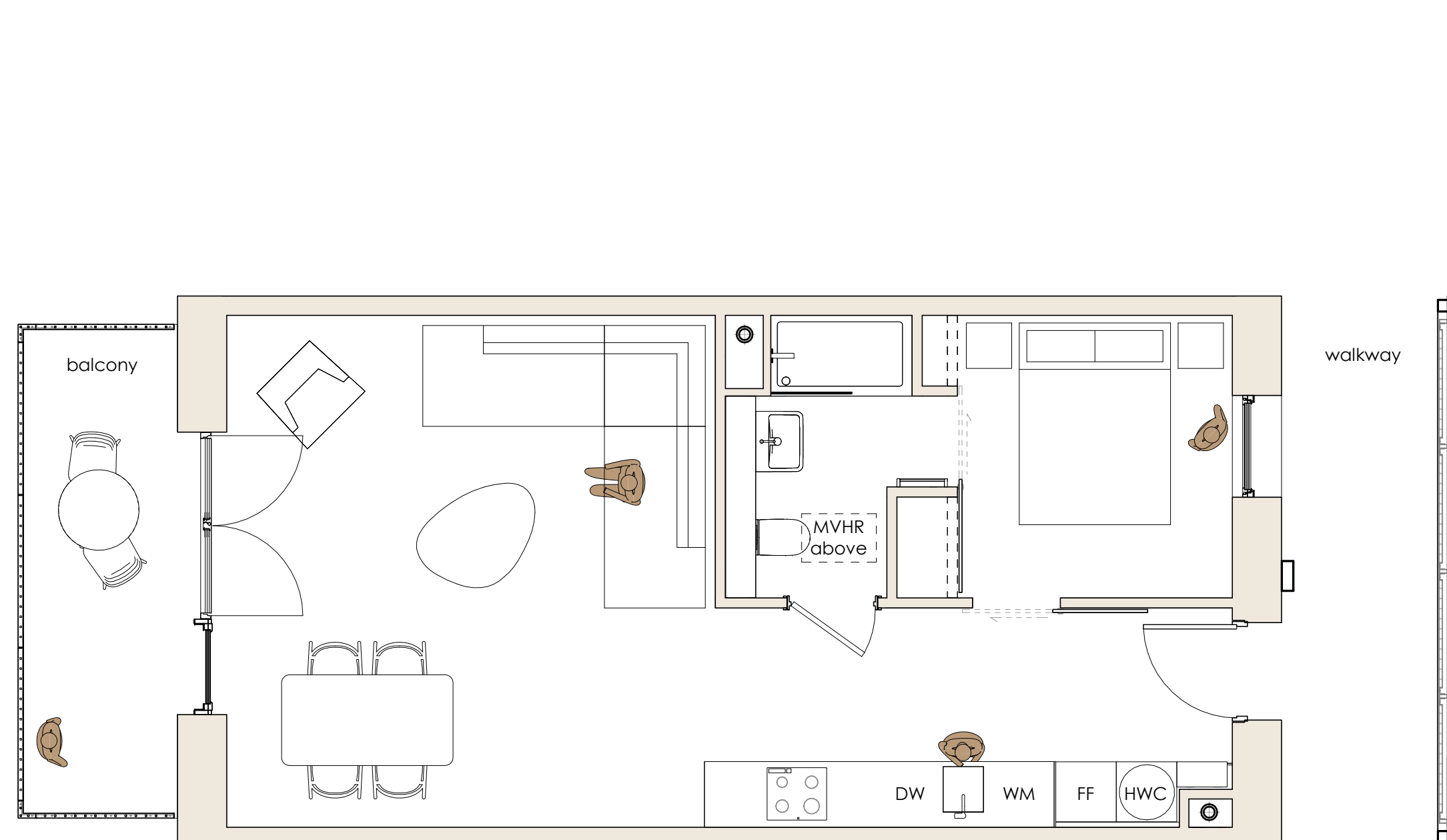
PLAN 1:50
